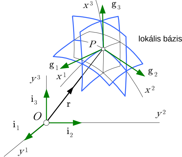
1.4. ábra. Görbevonallú KR
