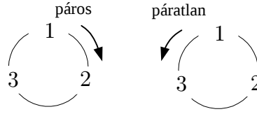
1.3. ábra. Páros és páratlan permutációk
