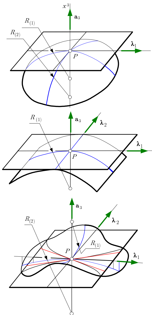
9.5. ábra. Elliptikus, parabolikus és hiperbolikus pontok a felületen
