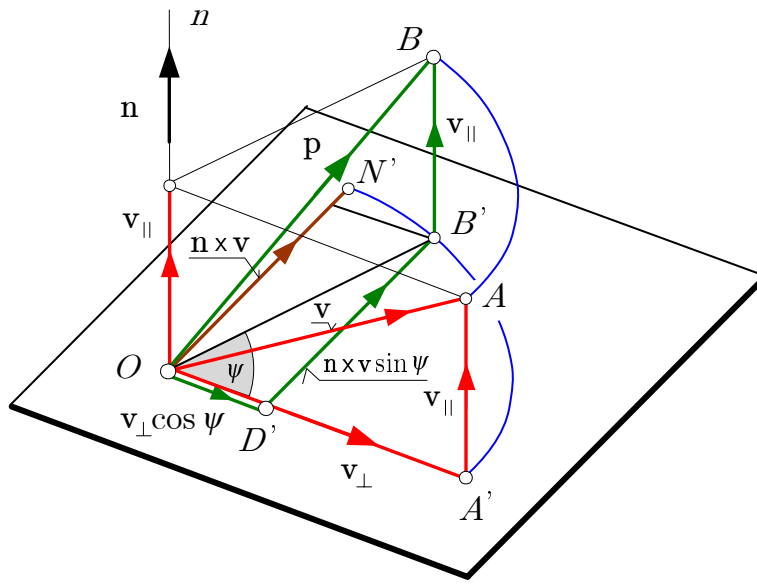
7.2. ábra. Véges forgatás
